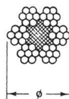
FUNE A 42 FILI E 1 ANIMA IN FIBRA TESSILE FORMAZIONE: A + 6 (1+6)
