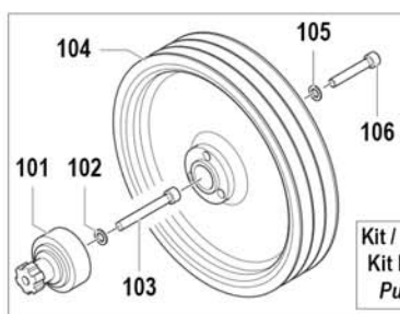
► 107 Kit / Optional Kit Puleggia Pulley Kit
